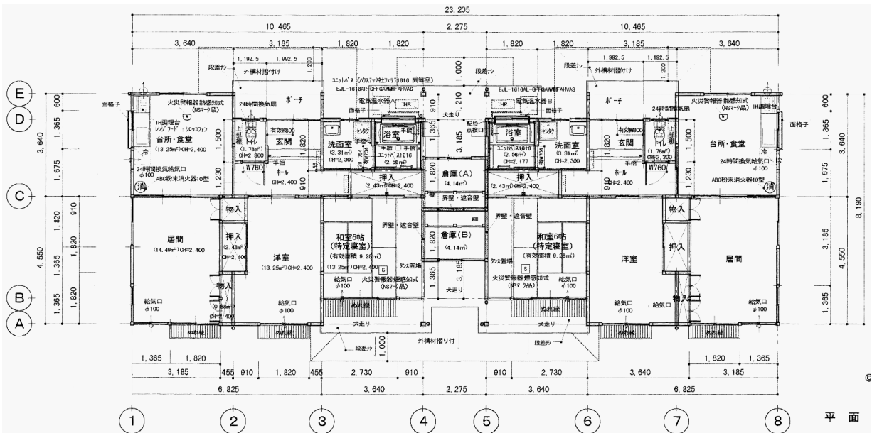
平面図
