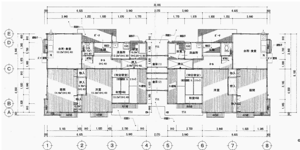
平面図
