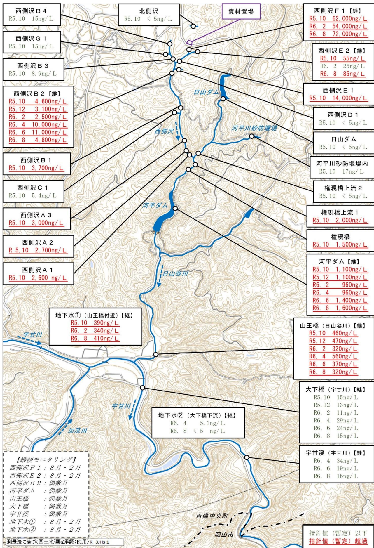
図－5 公共用水域及び地下水の調査地点及び結果
